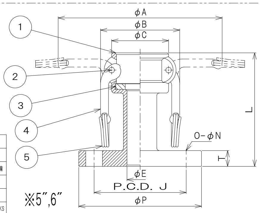
633-LBS SST サイズ別寸法表(単位 : mm)
